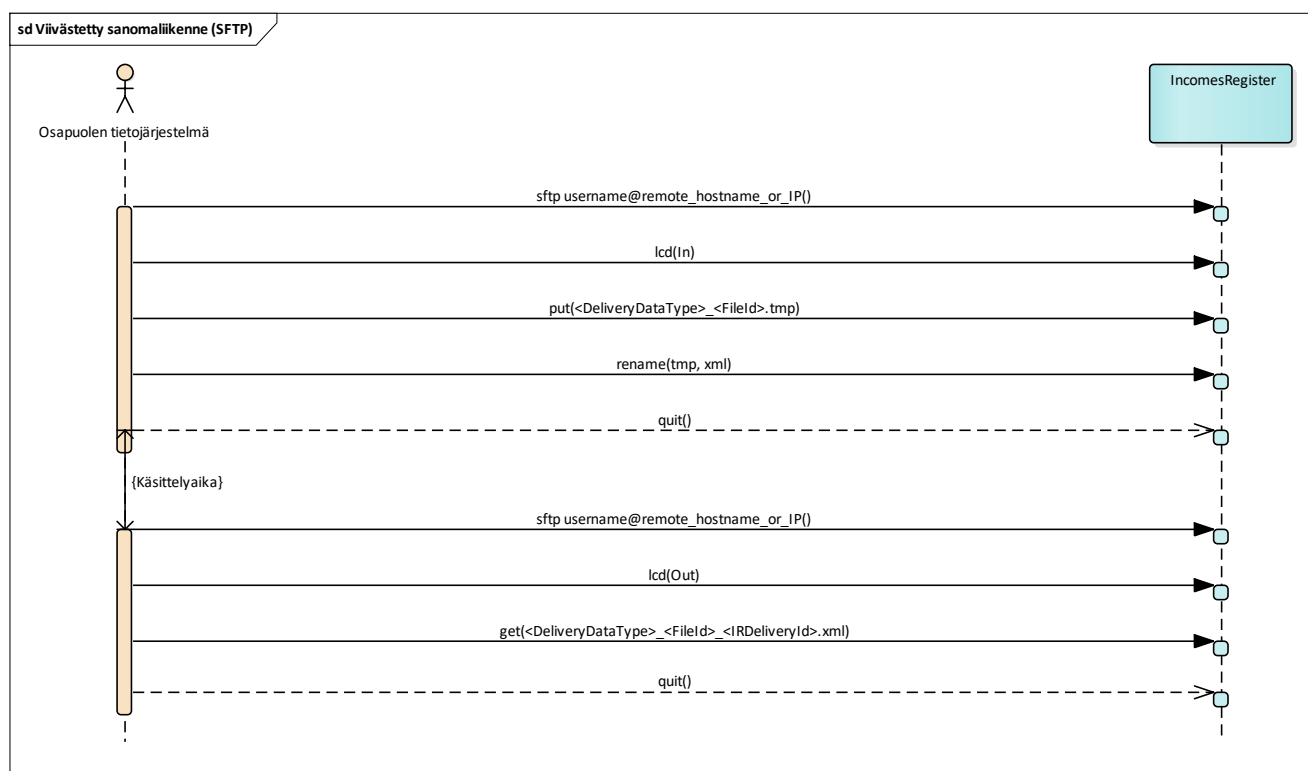
Bild 5. Sekvensschema för SFTP-kanalens kommunikationsmodell.
