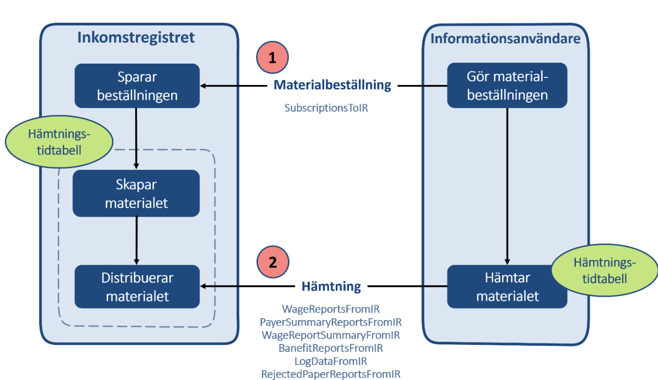
Bild 3. Datadistribution genom SFTP-gränssnittet.
