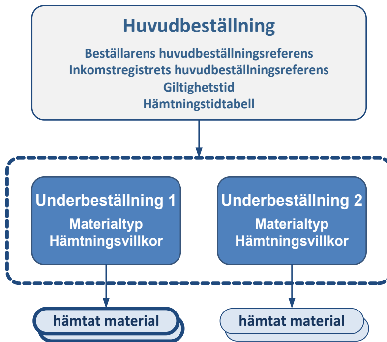
Bild 7. Struktur av materialbeställningar
