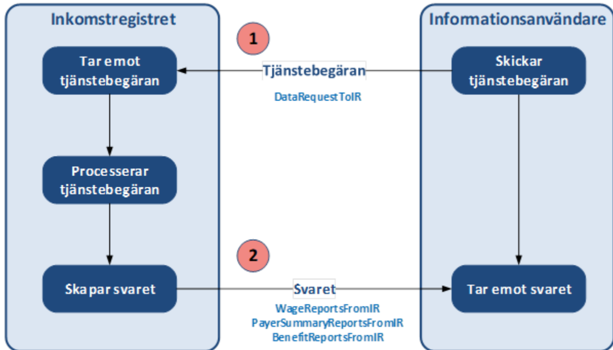
Bild 4. Datadistribution genom Web Service-gränssnittet i realtid.
