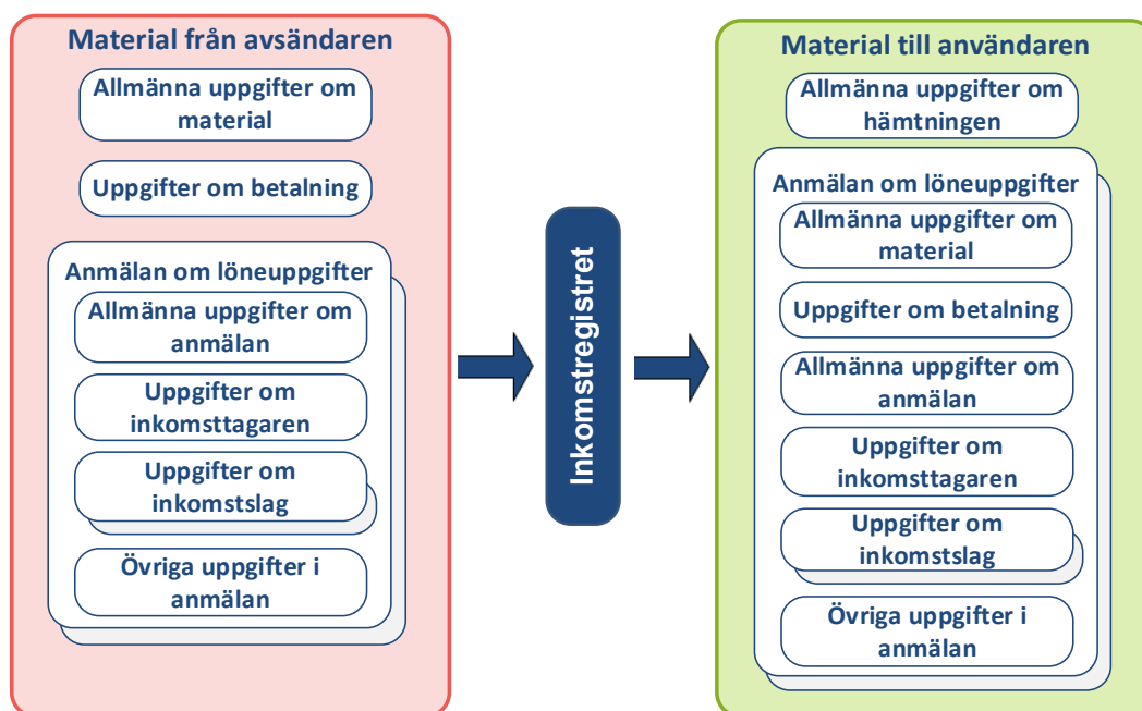
Bild 2. Allmän struktur av material som innehåller anmälningar om löneuppgifter.
