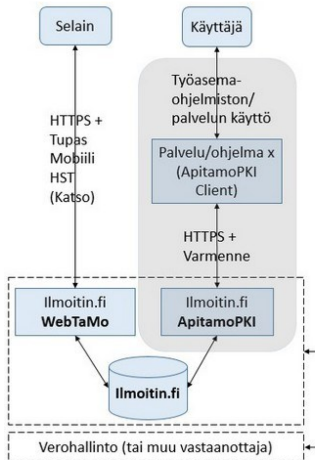
Kuva 1. Ilmoitin.fi-palvelukokonaisuus ja ApitamoPKI
